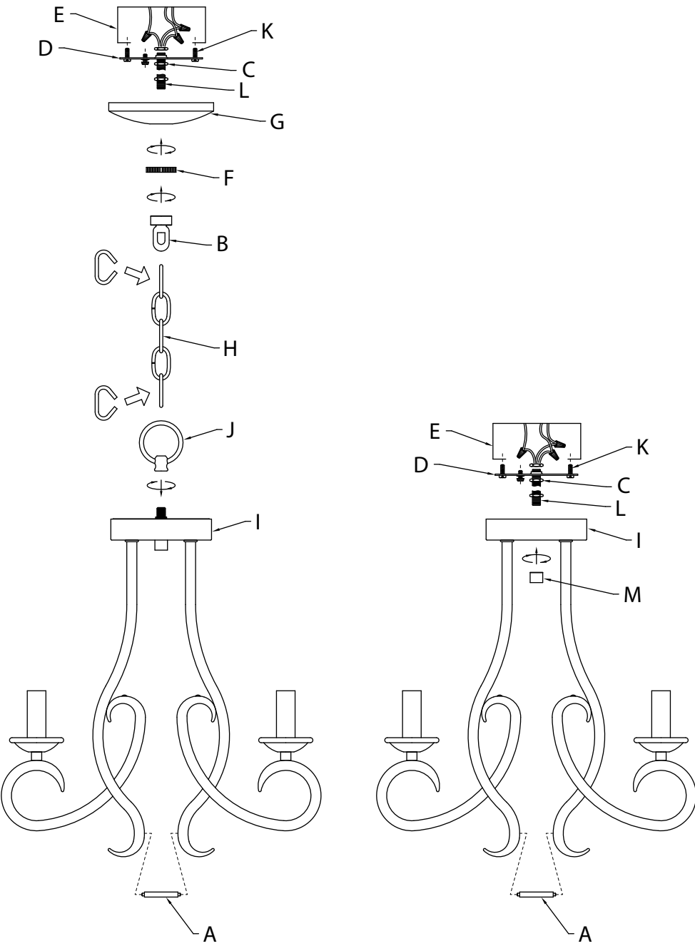
MONTAJE CON CADENA COLGANTE
