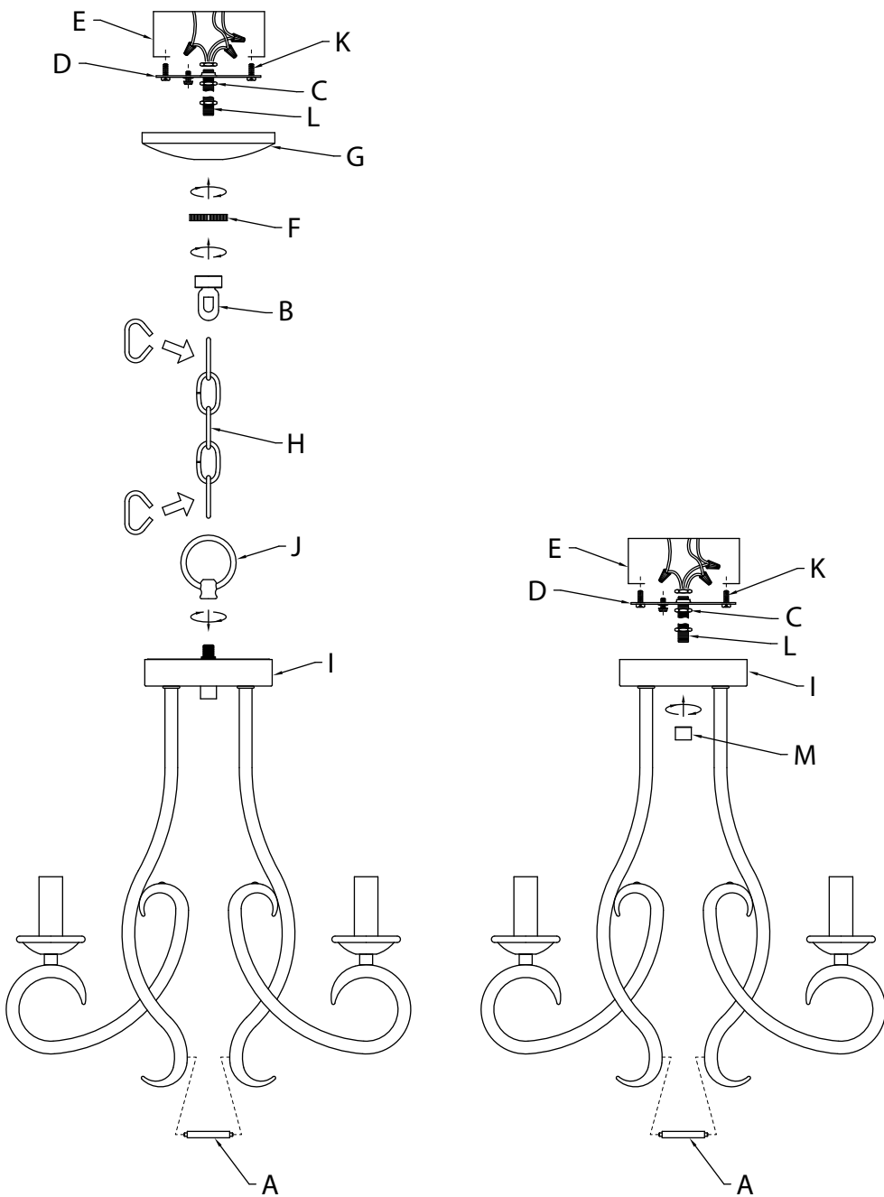
MONTAGE SUSPENDU AVEC CHAÎNE
